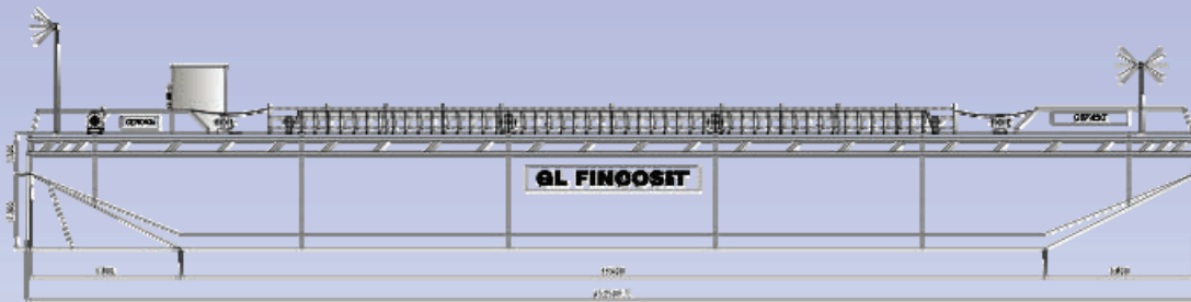
VISTA LONGITUDINALE
